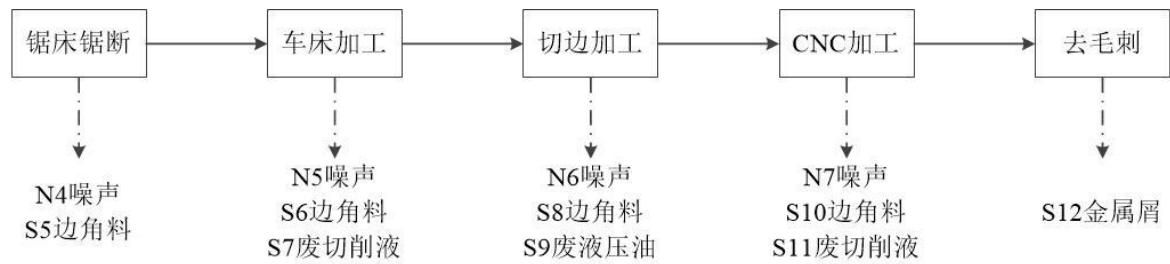
图 5.1-2 配套壳体加工工艺流程图
