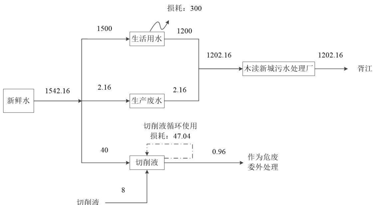
图 5.2 项目水平衡图 (单位: t/a)
