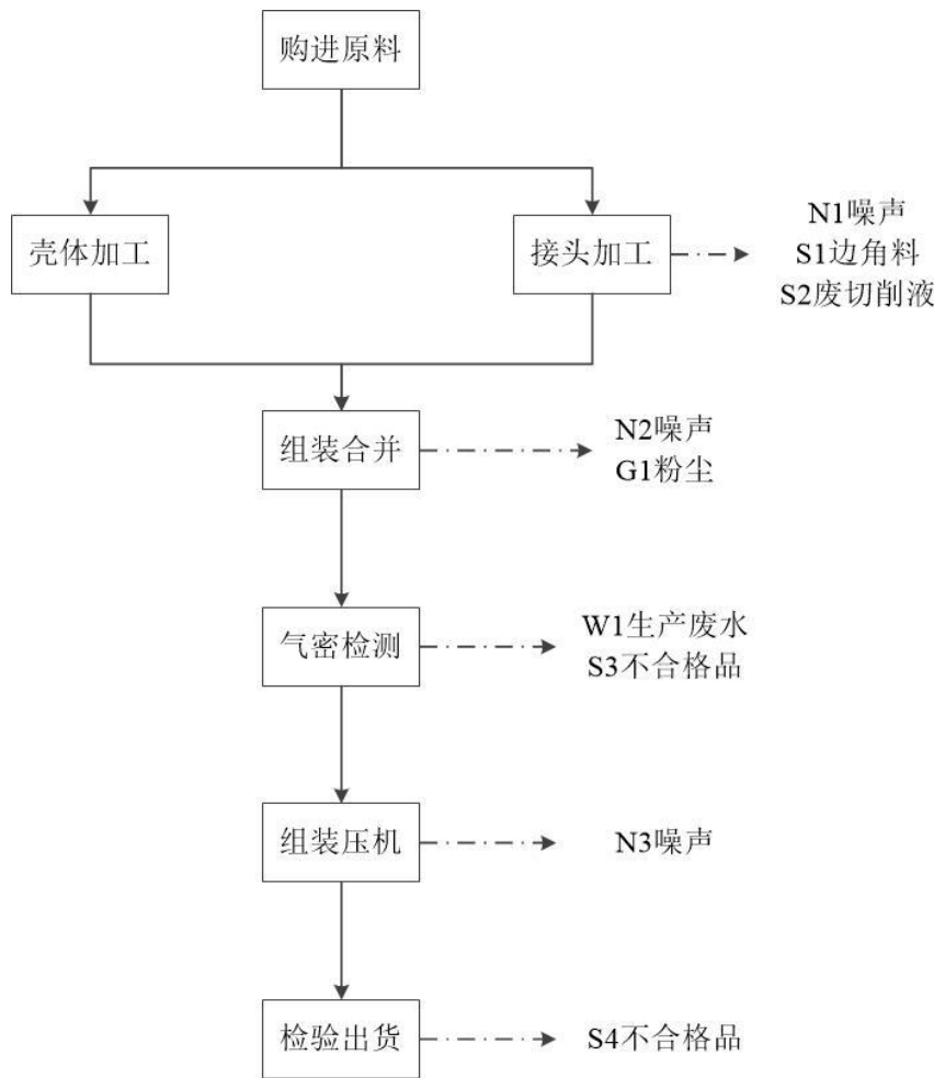
图 5.1-1 汽车空调配件工艺流程图
