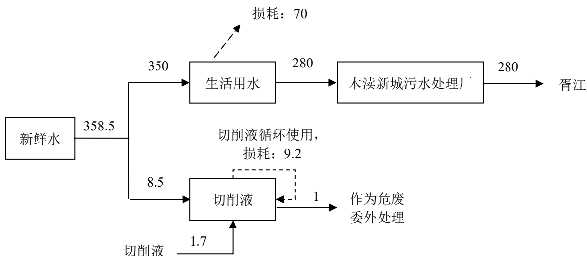
图 5-2 项目水平衡图 (单位: t/a)
