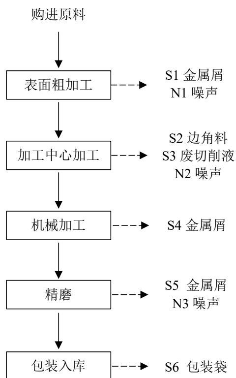
图 5-1 工艺流程图
