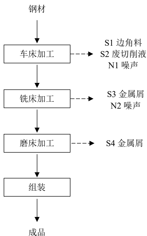
图 1-1 原有项目生产工艺流程图
