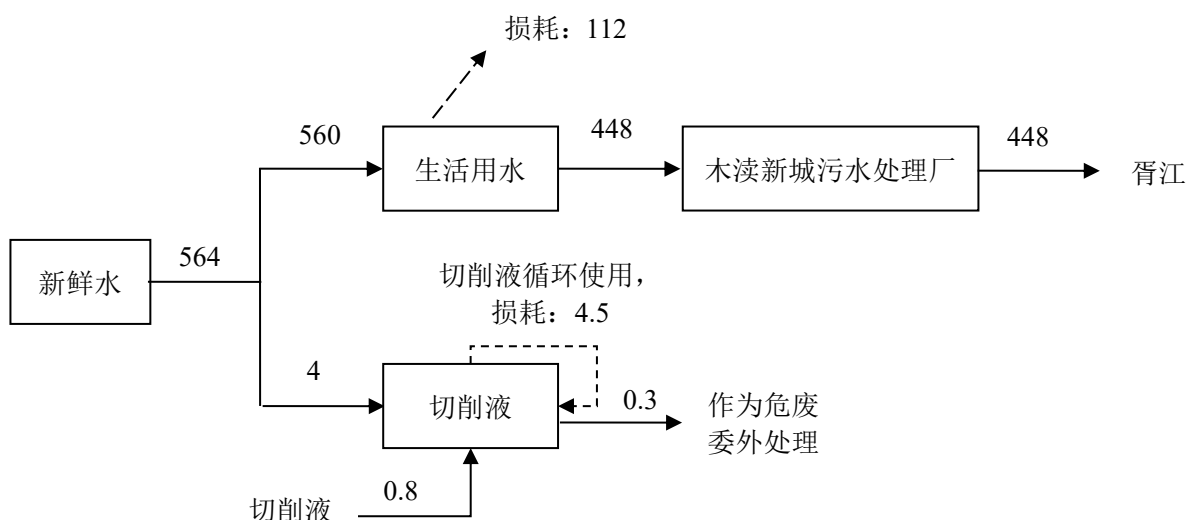
图 1-2 现有项目水平衡图（单位：t/a）
