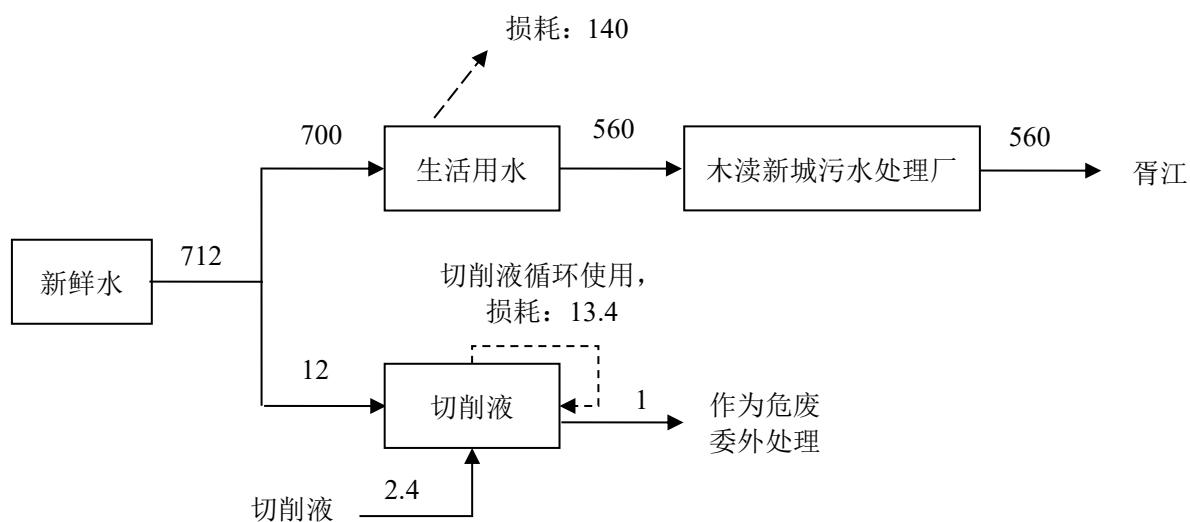
图 5-3 扩建后全厂水平衡图 (单位: t/a)
