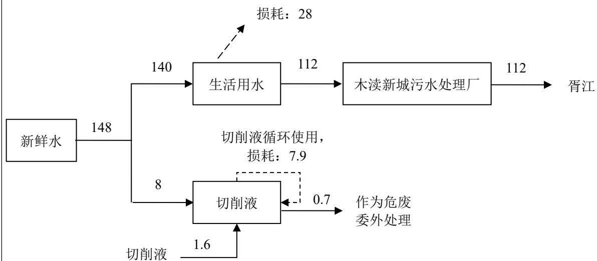
图 5-2 扩建项目水平衡图 (单位: t/a)
