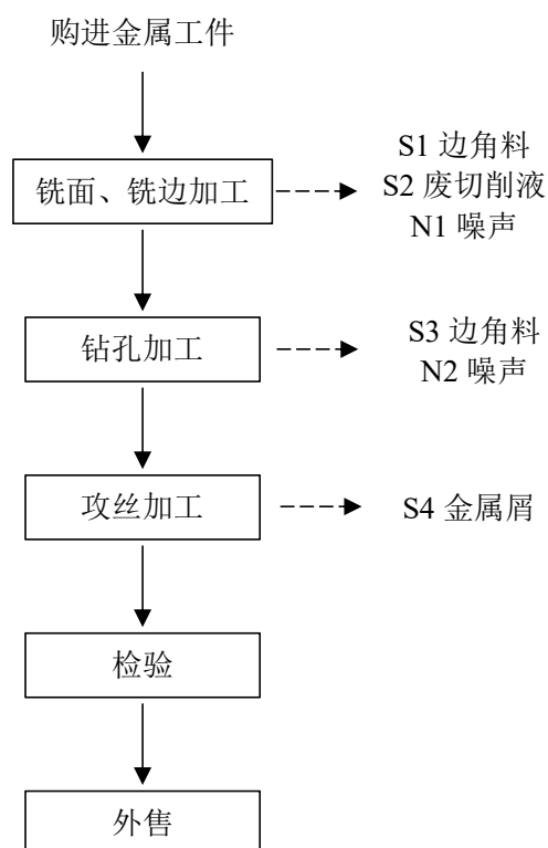
图 1-1 现有项目工艺流程图
