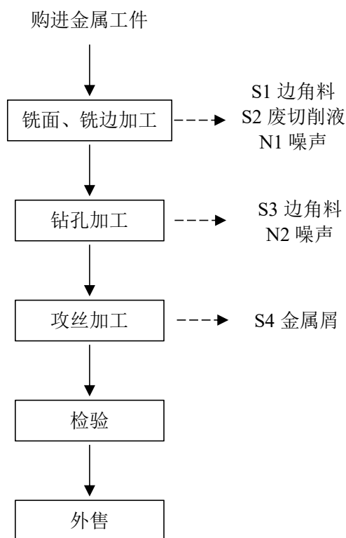
图 5-1 工艺流程图
